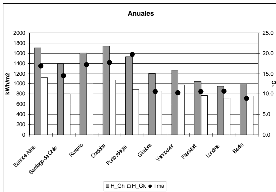
Figura 4: Temperaturas medias anuales y disponibilidad de radiación global anual.
