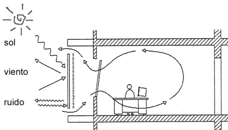
Figura1: Esquema conceptual de una DF. (Nolte y Pasquay, 1997)
